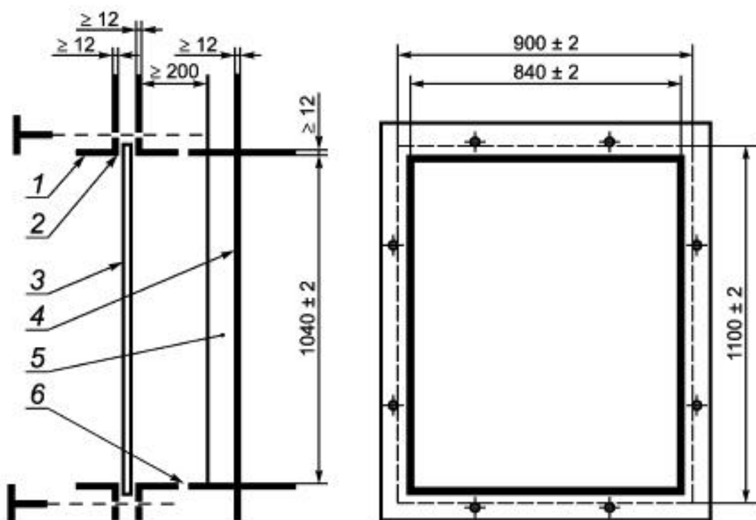
Рисунок 4 - Стальная рама для крепления образца
