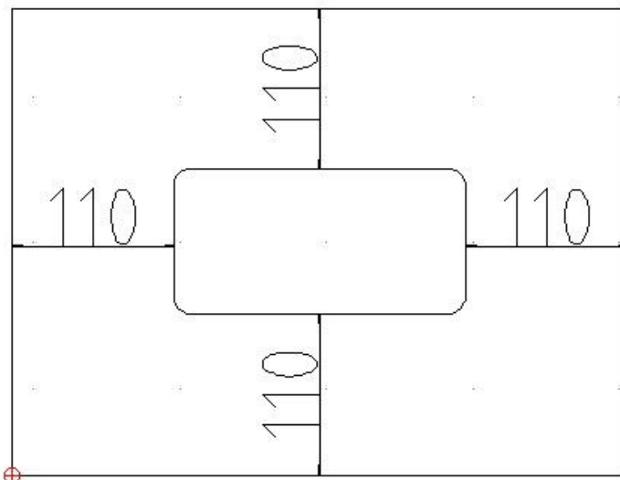
Внутренний вырез
